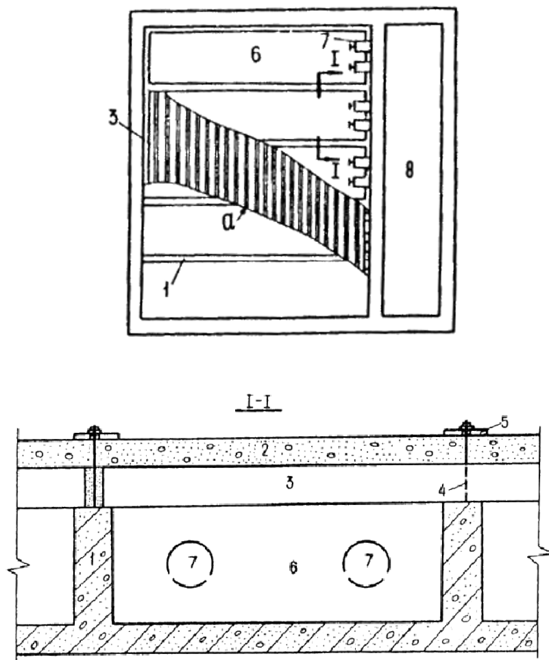
Черт.29. Дренаж из монолитного полимербетона
