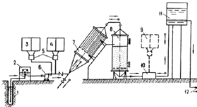
Черт.43. Принципиальная схема обезжелезивания, обезфторивания, и умягчения воды на установках типа "Струя"
