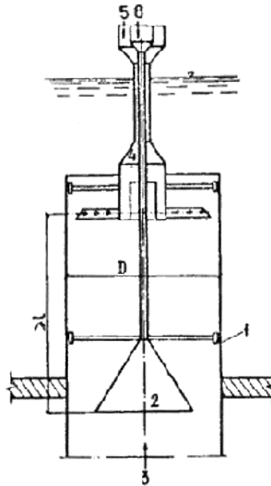
Черт.6. Схема совмещения диффузорного и камерно-лучевого распределителей
