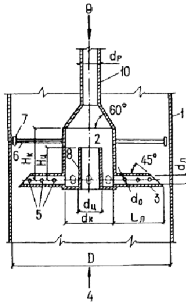
Черт.3. Камерно-лучевой распределитель (тип II, расположение - внутри трубопровода)
