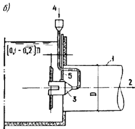
Черт.4. Схемы установки камерно-лучевых распределителей (тип II)
