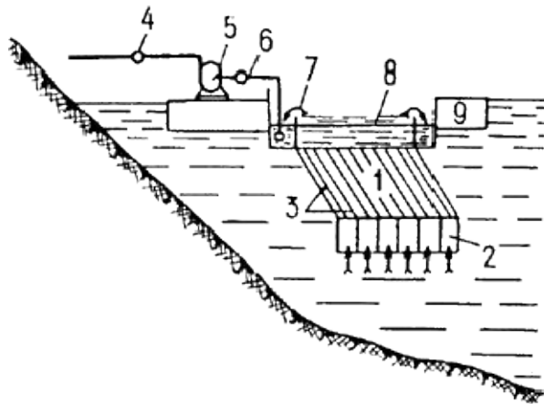
Черт.34. Плавающий водозабор-осветлитель
