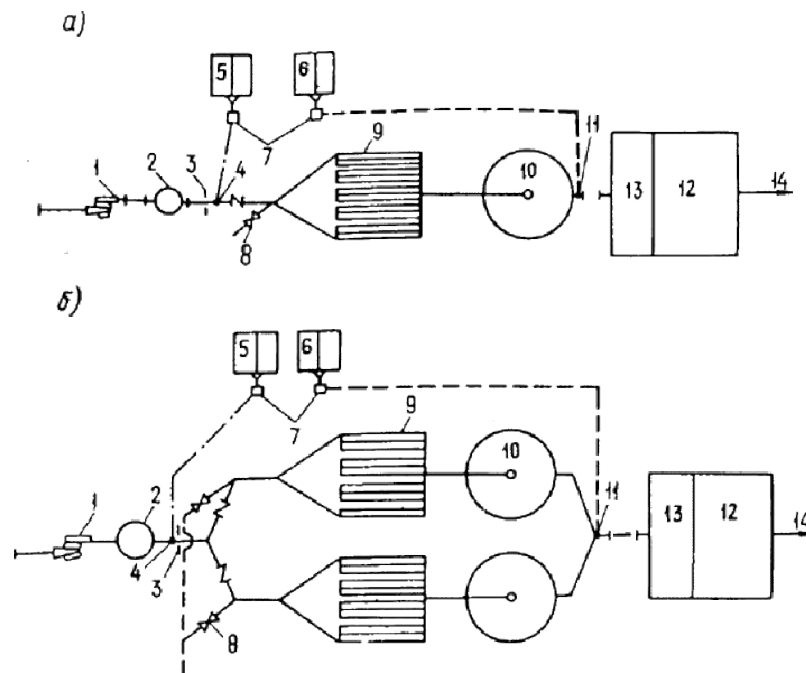
Черт.42. Принципиальная схема работы установок типа "Струя"
